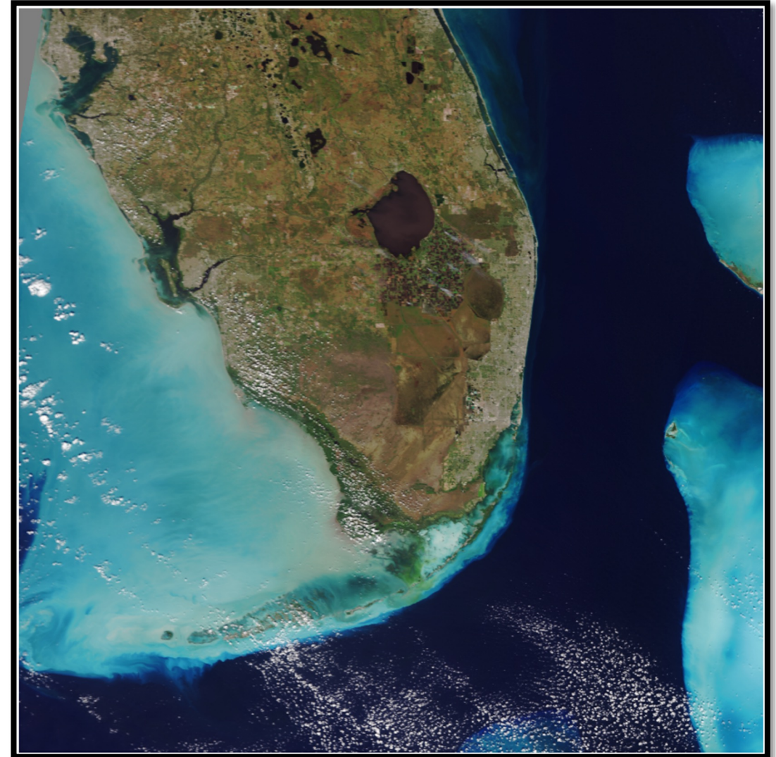
S-NPP VIIRS True Color Imagery
